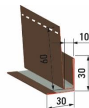
Narożnik bezwkrętowy zew / wew
