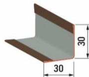
Narożnik wew / zew
