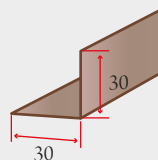
Narożnik wewnętrzny
